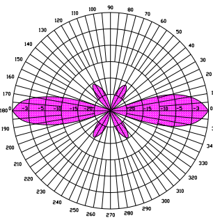
垂直方向图
