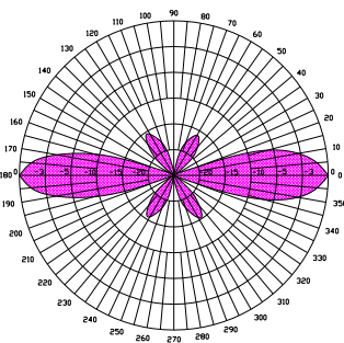
垂直方向图
