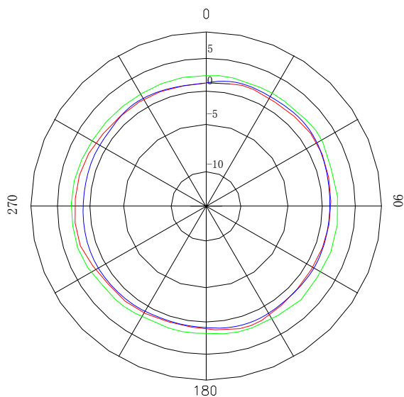
水平面方向图 (2. 4G天线) Horizontal Pattern
