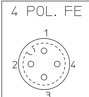
OBUDOWA ZENSKA 4 POLOWA WIDOK OD STRONY DRUTOW FEMALE INSERT 4P VIEW FROM WIRES SIDE
