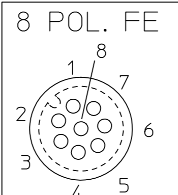
OBUDOWA ZENSKA 8 POLOWA WIDOK OD STRONY DRUTOW FEMALE INSERT 8P VIEW FROM WIRES SIDE
