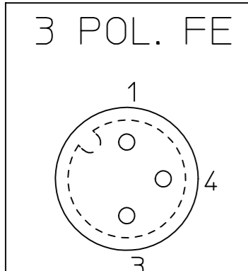
OBUDOWA ZENSKA 3 POLOWA WIDOK OD STRONY DRUTOW FEMALE INSERT 3P VIEW FROM WIRES SIDE
