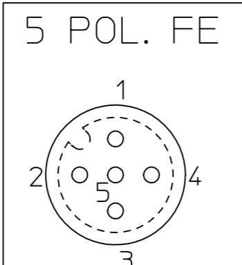
OBUDOWA ZENSKA 5 POLOWA WIDOK OD STRONY DRUTOW FEMALE INSERT 5P VIEW FROM WIRES SIDE
