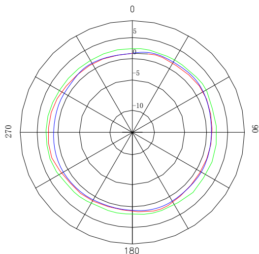
水平面方向图(2.4G天线) Horizontal Pattern
